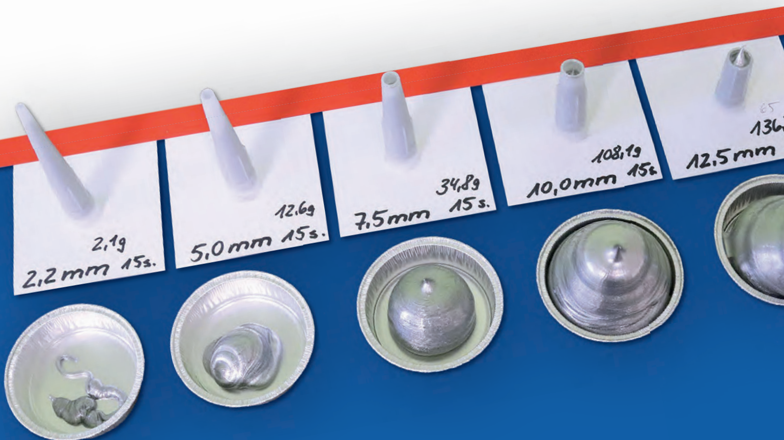
Austragsmenge bei verschiedenen großen Düsenöffnungen
