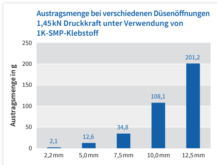
Austragsmenge bei verschiedenen großen Düsenöffnungen
